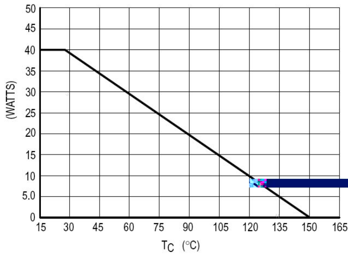
P_D - T_C
